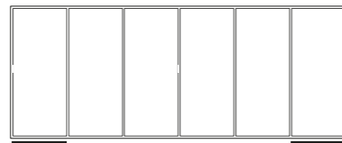
6 vantaux / 3 rails
